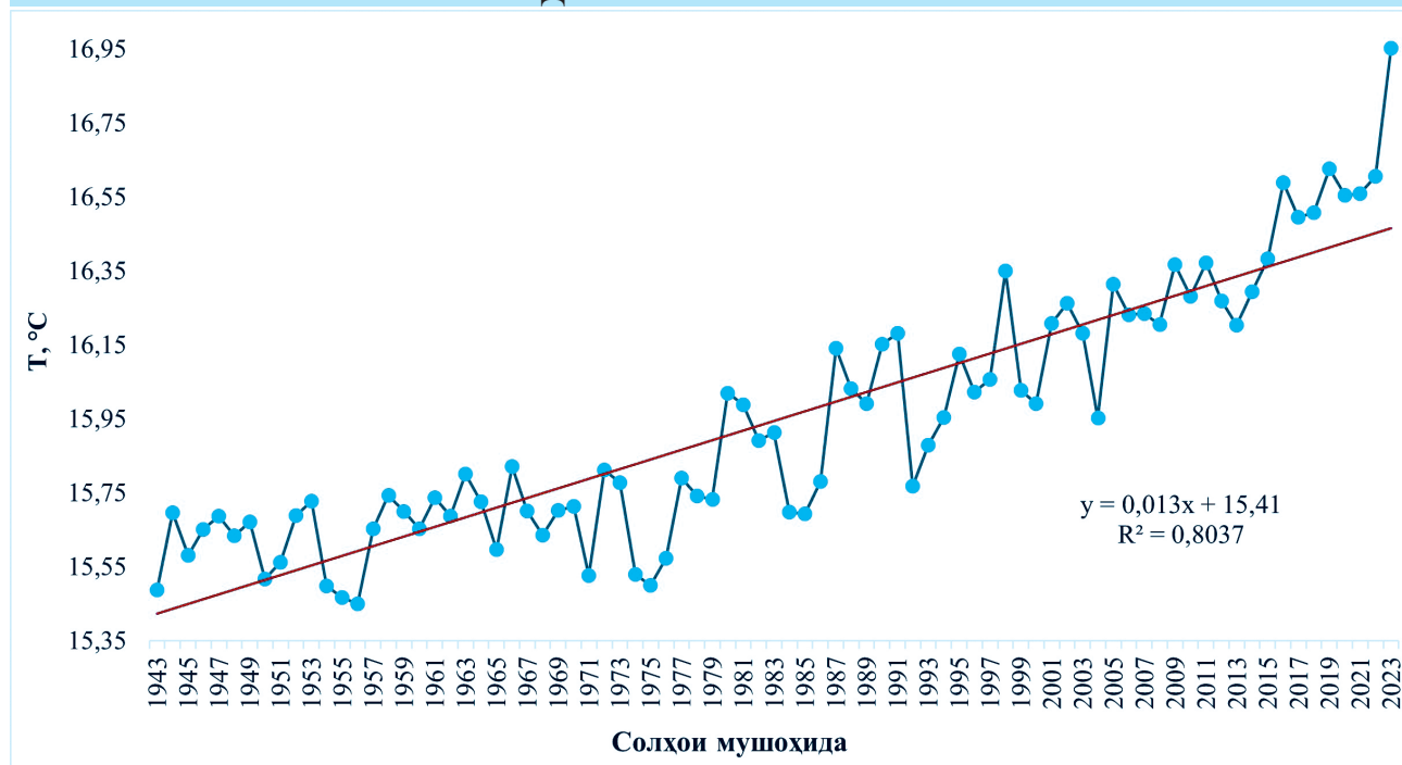
Ҳарорати миёнаи ҷаҳонӣ ( ^\circ\text{C} ) дар моҳҳои июли солҳои 1943-2023
